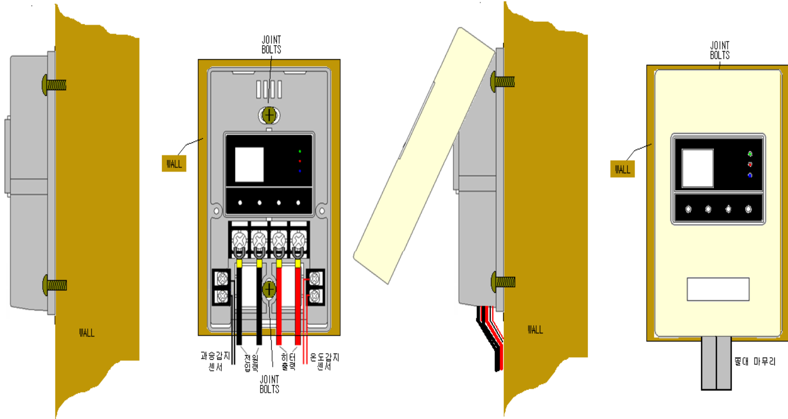
시공결선방법 #1
